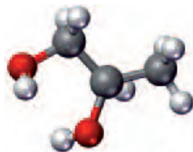
Propylène glycol C 3 H 8 O 2
