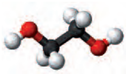
Ethylène glycol C 2 H 6 O 2
